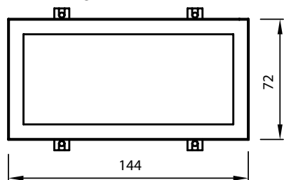
Maattekening A
